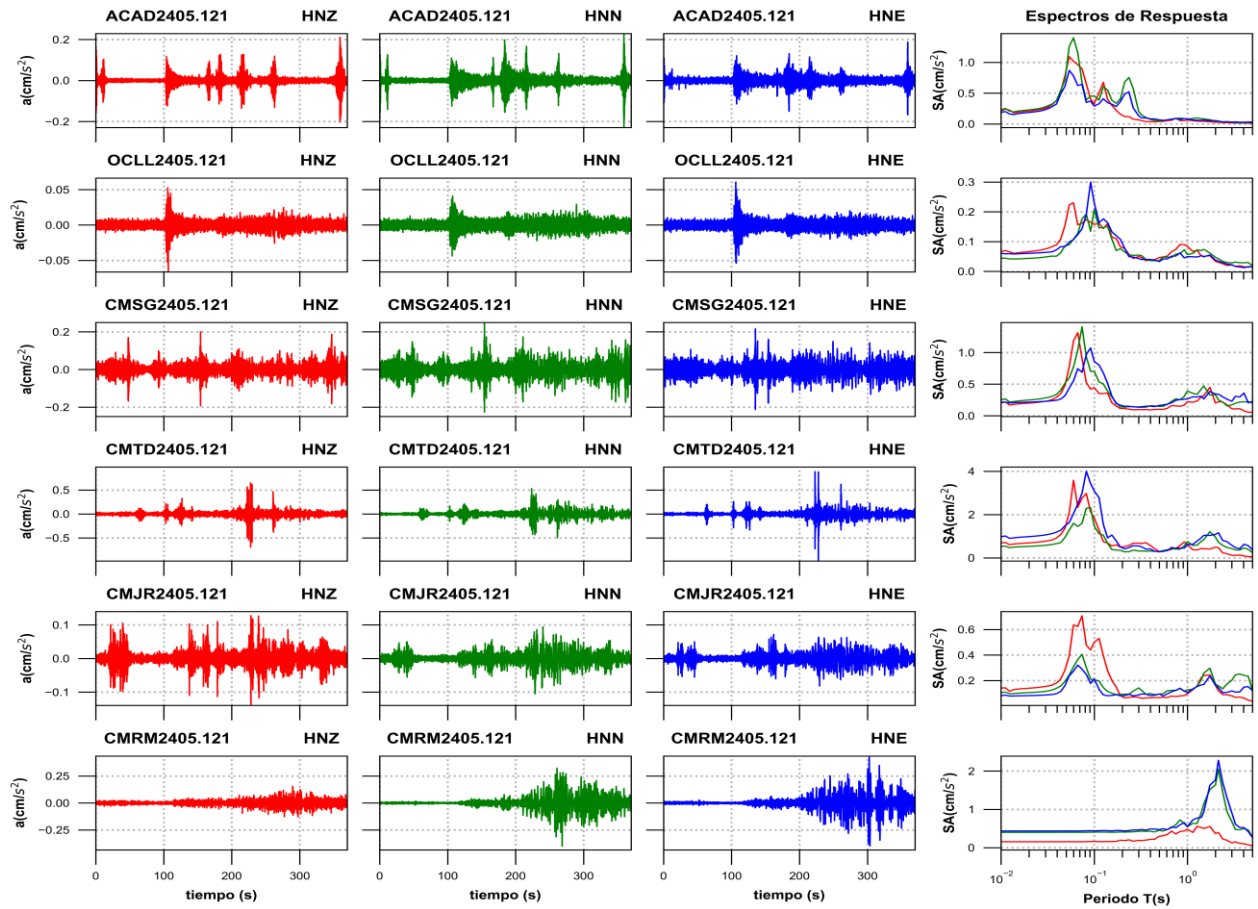
Figura 3c. Acelerogramas registrados y espectros de respuesta estimados para los registros obtenidos durante el sismo del 12 de mayo de 2024 (M6.6)
