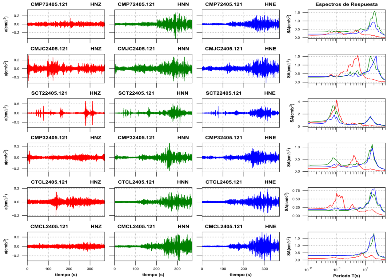
Figura 3f. Acelerogramas registrados y espectros de respuesta estimados para los registros obtenidos durante el sismo del 12 de mayo de 2024 (M6.6)
