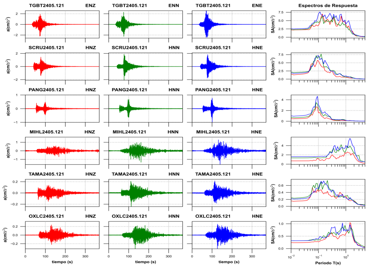
Figura 3a. Acelerogramas registrados y espectros de respuesta estimados para los registros obtenidos durante el sismo del 12 de mayo de 2024 (M6.6)
