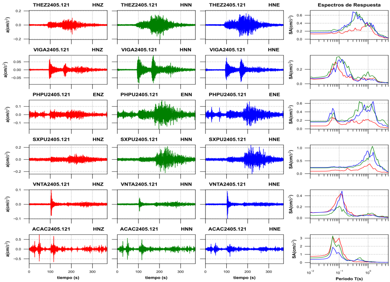
Figura 3b. Acelerogramas registrados y espectros de respuesta estimados para los registros obtenidos durante el sismo del 12 de mayo de 2024 (M6.6)
