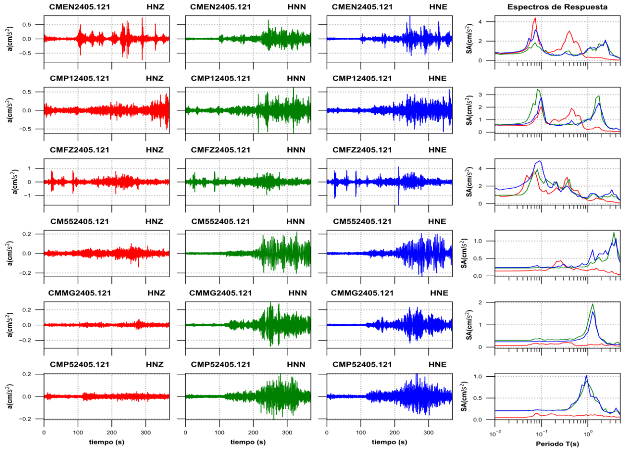
Figura 3d. Acelerogramas registrados y espectros de respuesta estimados para los registros obtenidos durante el sismo del 12 de mayo de 2024 (M6.6)
