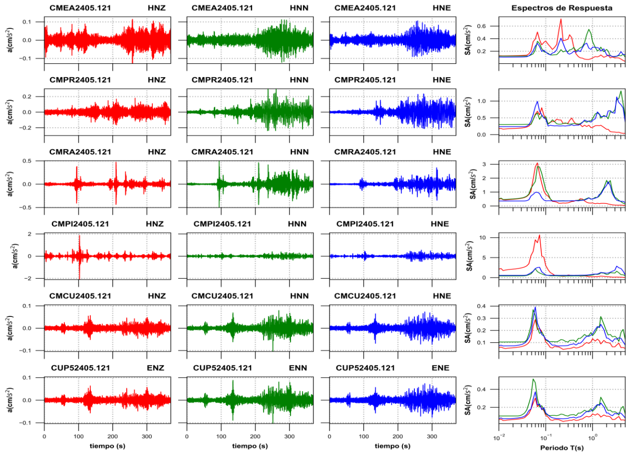
Figura 3e. Acelerogramas registrados y espectros de respuesta estimados para los registros obtenidos durante el sismo del 12 de mayo de 2024 (M6.6)
