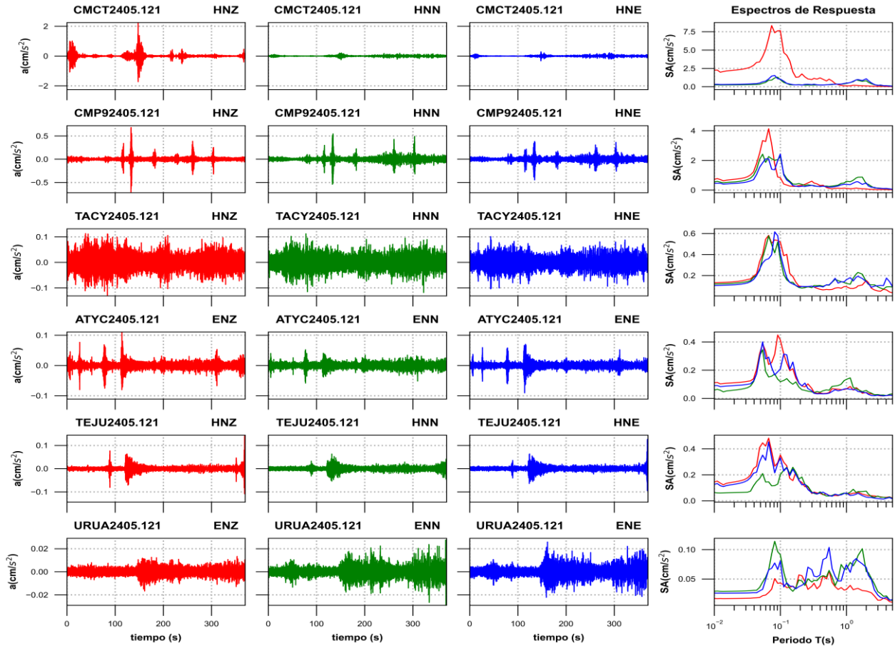
Figura 3g. Acelerogramas registrados y espectros de respuesta estimados para los registros obtenidos durante el sismo del 12 de mayo de 2024 (M6.6)
