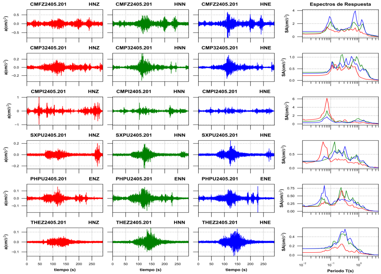
Figura 3f. Acelerogramas registrados y espectros de respuesta estimados para los registros obtenidos durante el sismo del 20 de mayo de 2024 (M4.9)
