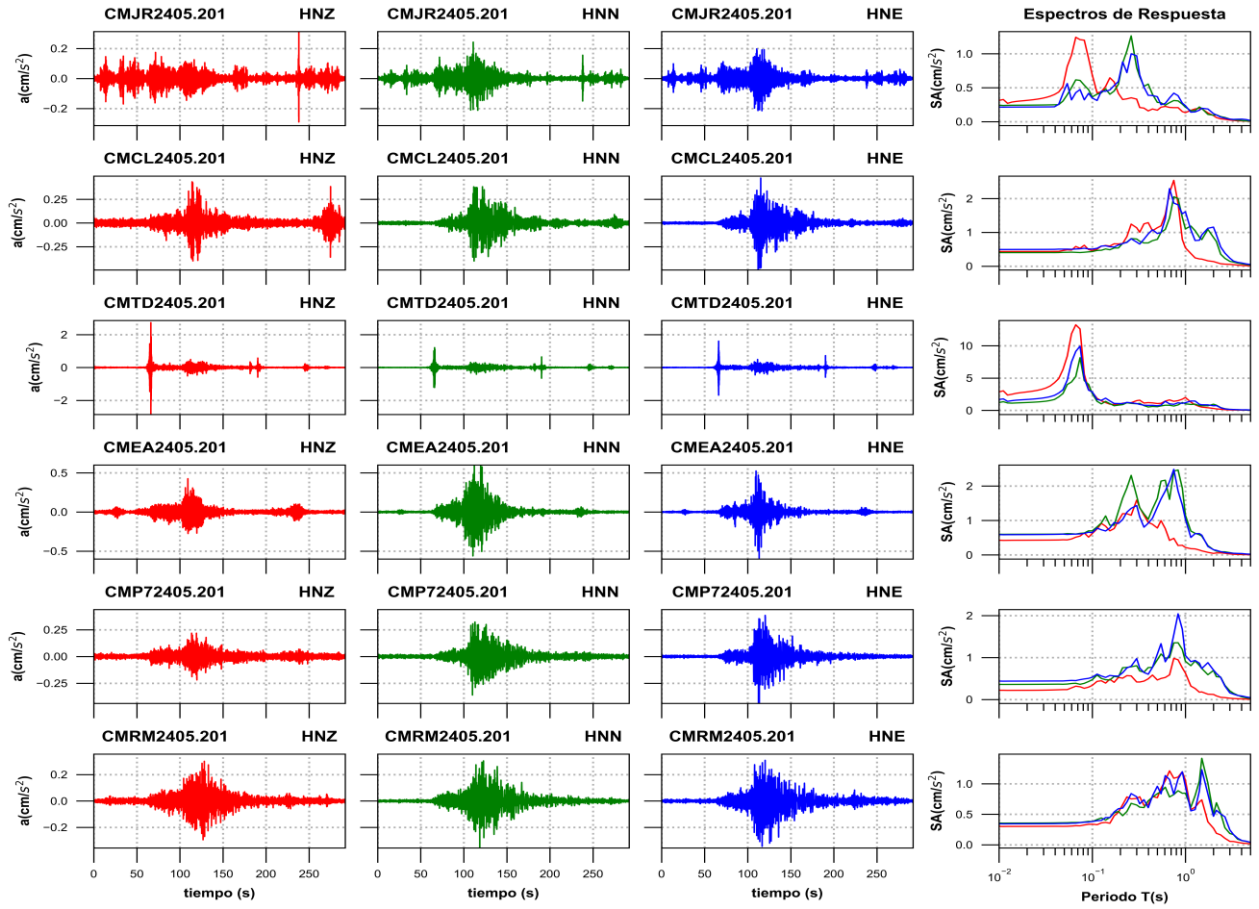
Figura 3d. Acelerogramas registrados y espectros de respuesta estimados para los registros obtenidos durante el sismo del 20 de mayo de 2024 (M4.9)
