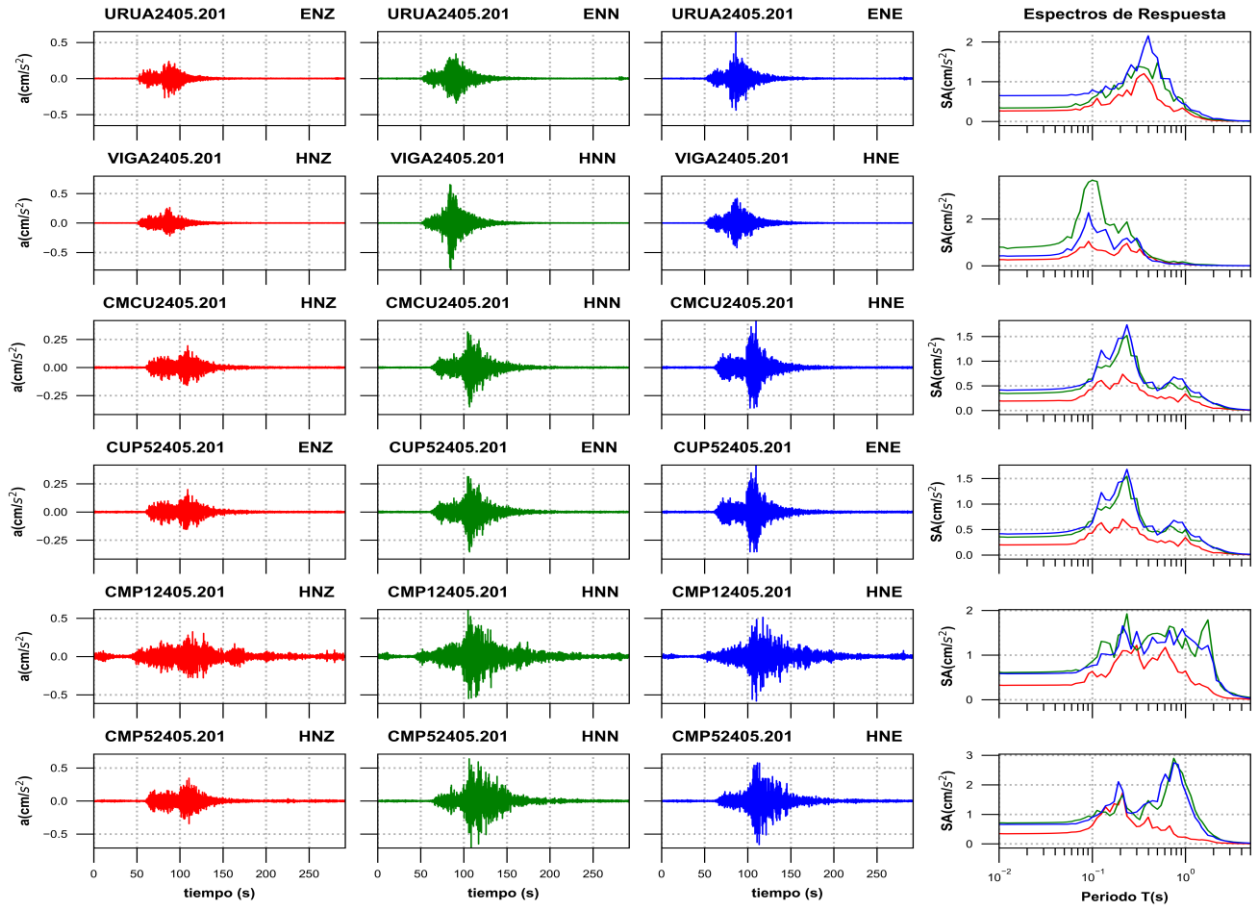
Figura 3b. Acelerogramas registrados y espectros de respuesta estimados para los registros obtenidos durante el sismo del 20 de mayo de 2024 (M4.9)
