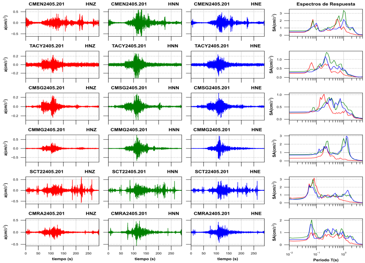
Figura 3c. Acelerogramas registrados y espectros de respuesta estimados para los registros obtenidos durante el sismo del 20 de mayo de 2024 (M4.9)
