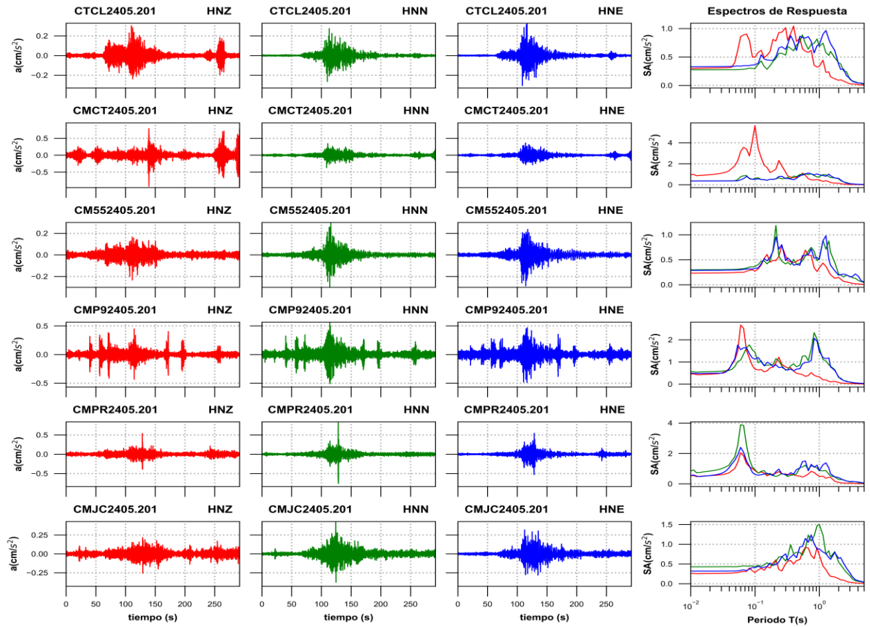
Figura 3e. Acelerogramas registrados y espectros de respuesta estimados para los registros obtenidos durante el sismo del 20 de mayo de 2024 (M4.9)
