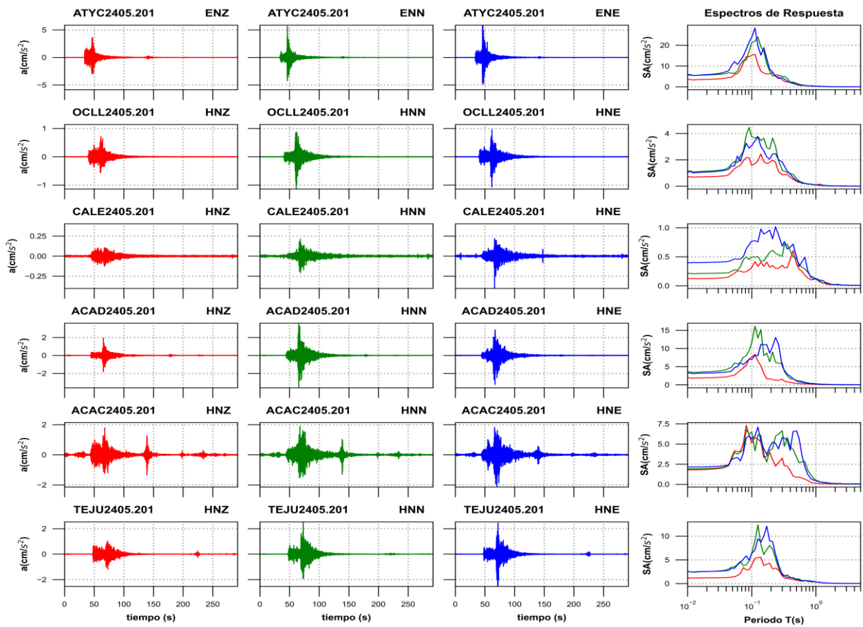
Figura 3a. Acelerogramas registrados y espectros de respuesta estimados para los registros obtenidos durante el sismo del 20 de mayo de 2024 (M4.9)
