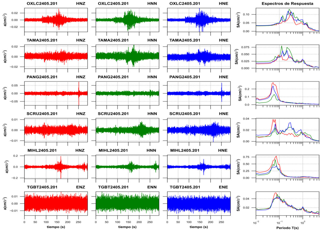
Figura 3g. Acelerogramas registrados y espectros de respuesta estimados para los registros obtenidos durante el sismo del 20 de mayo de 2024 (M4.9)
