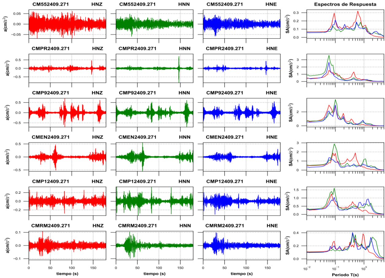
Figura 3d. Acelerogramas registrados y espectros de respuesta estimados para los registros obtenidos durante el sismo del 26 de septiembre de 2024 (M2.7)
