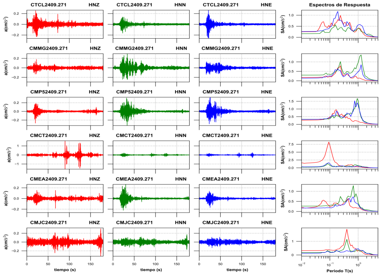
Figura 3c. Acelerogramas registrados y espectros de respuesta estimados para los registros obtenidos durante el sismo del 26 de septiembre de 2024 (M2.7)
