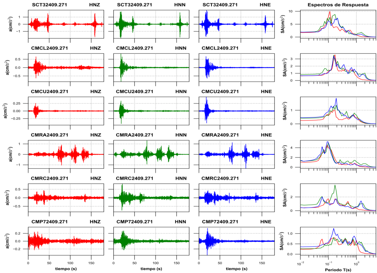
Figura 3b. Acelerogramas registrados y espectros de respuesta estimados para los registros obtenidos durante el sismo del 26 de septiembre de 2024 (M2.7)
