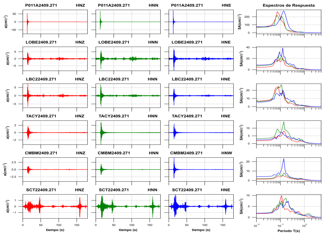
Figura 3a. Acelerogramas registrados y espectros de respuesta estimados para los registros obtenidos durante el sismo del 26 de septiembre de 2024 (M2.7)
