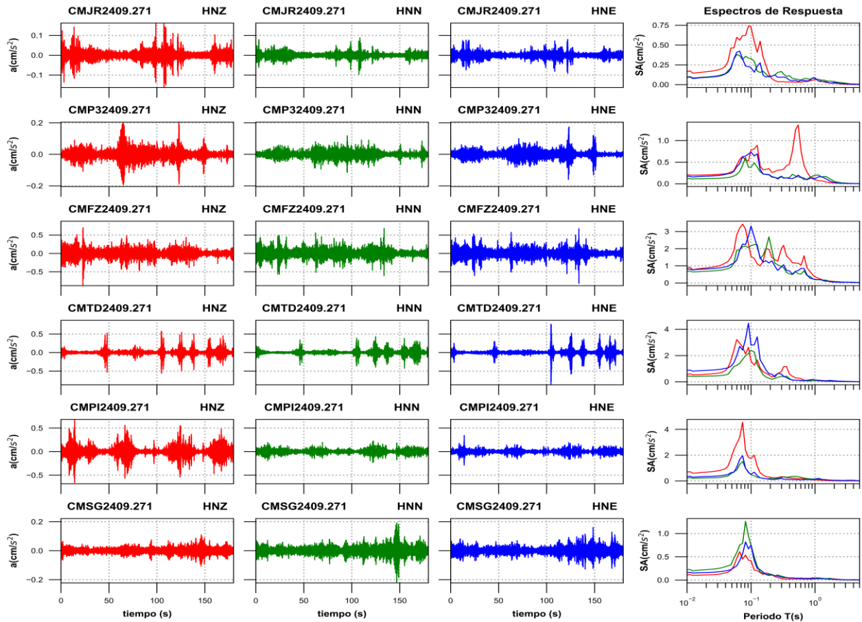
Figura 3e. Acelerogramas registrados y espectros de respuesta estimados para los registros obtenidos durante el sismo del 26 de septiembre de 2024 (M2.7)
