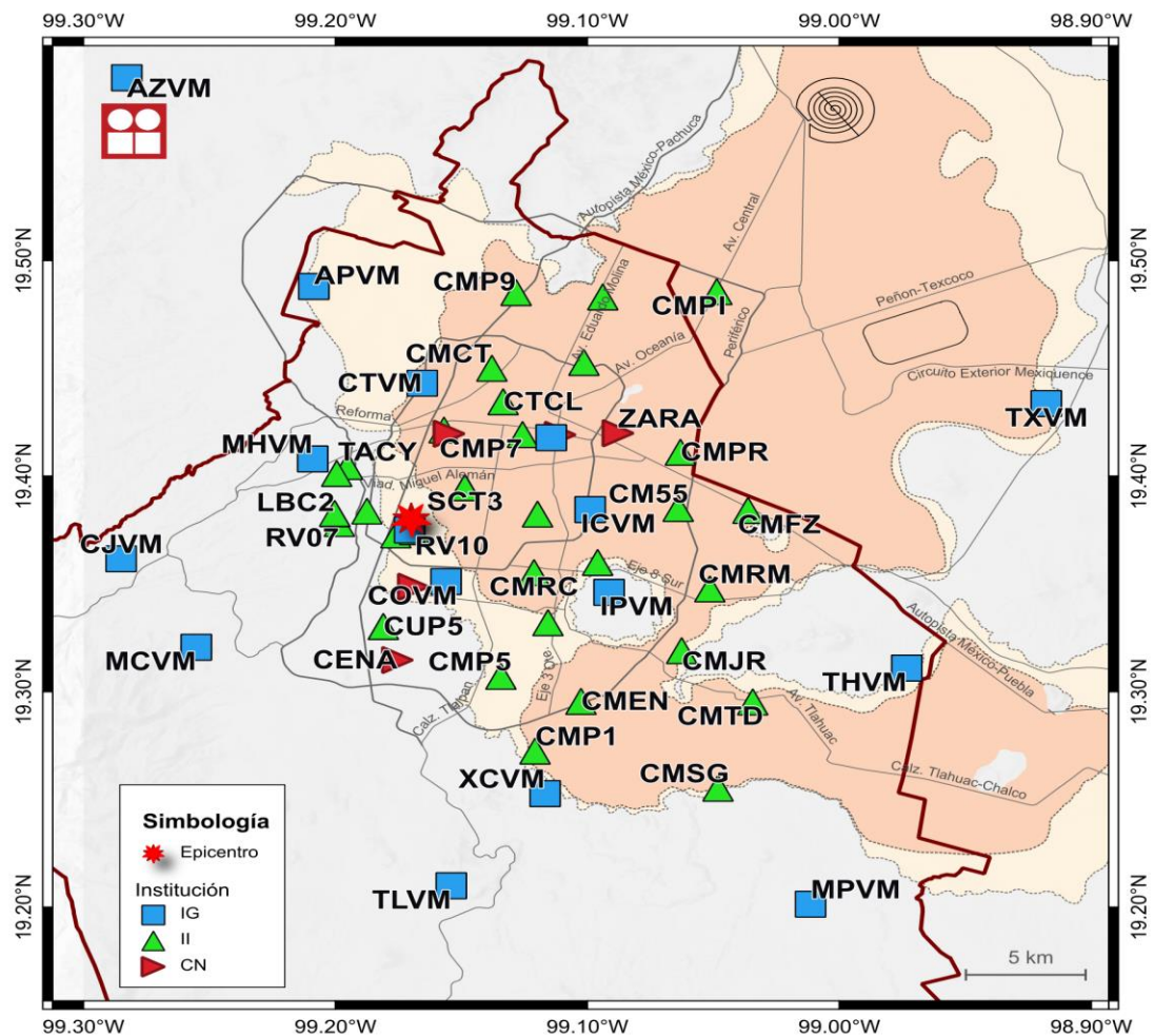
Figura 1. Epicentro del sismo del 15 de diciembre de 2024 (M2.2) y estaciones sísmicas empleadas en la elaboración del mapa preliminar de PGA. Las estaciones pertenecientes a la Red Acelerográfica del Instituto de Ingeniería de la UNAM (RAII-UNAM) son operadas por la Unidad de Instrumentación Sísmica. Las estaciones IG y CN mostradas son operadas por el Servicio Sismológico Nacional y el Centro Nacional de Prevención de Desastres, respectivamente.
