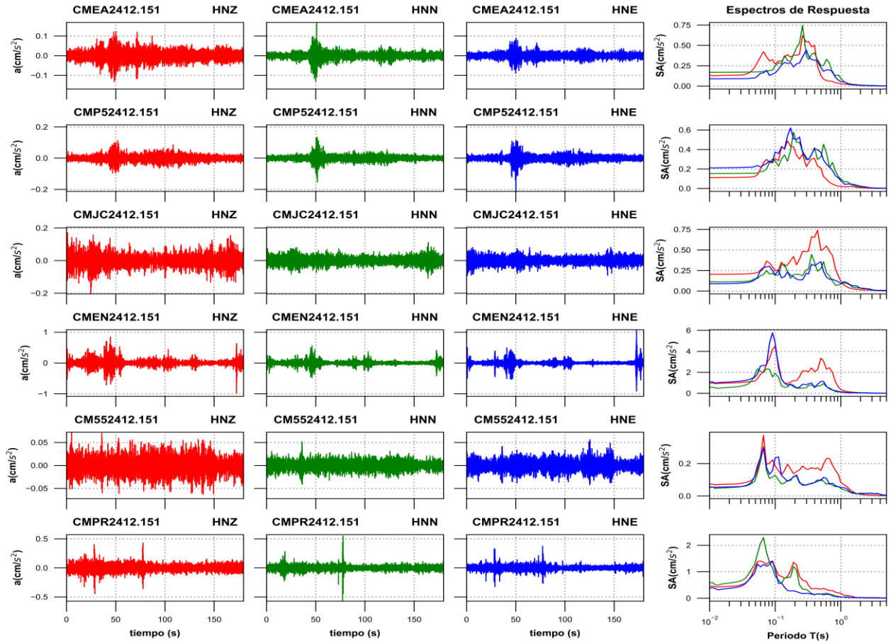
Figura 3d. Acelerogramas registrados y espectros de respuesta estimados para los registros obtenidos durante el sismo del 15 de diciembre de 2024 (M2.2)
