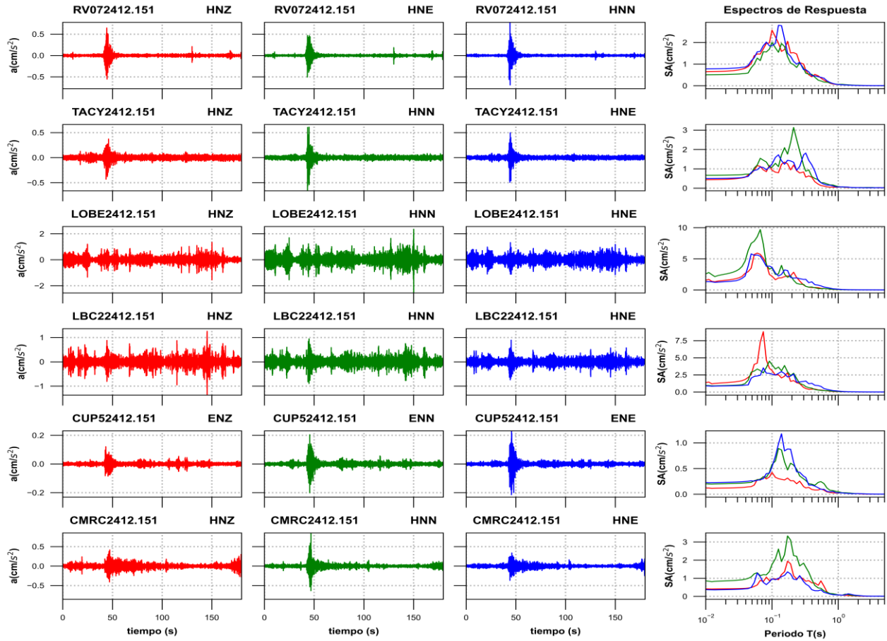
Figura 3b. Acelerogramas registrados y espectros de respuesta estimados para los registros obtenidos durante el sismo del 15 de diciembre de 2024 (M2.2)
