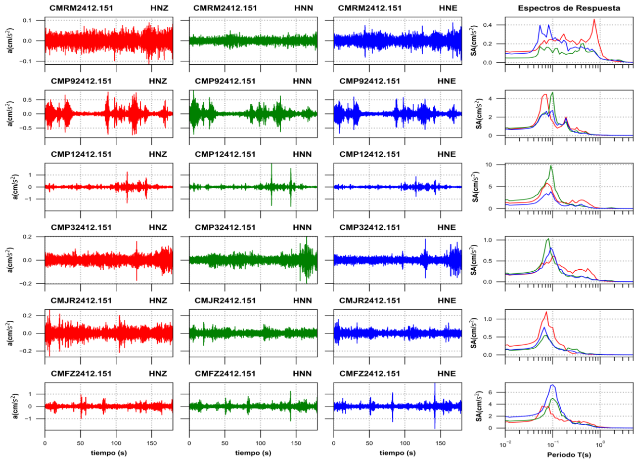
Figura 3e. Acelerogramas registrados y espectros de respuesta estimados para los registros obtenidos durante el sismo del 15 de diciembre de 2024 (M2.2)
