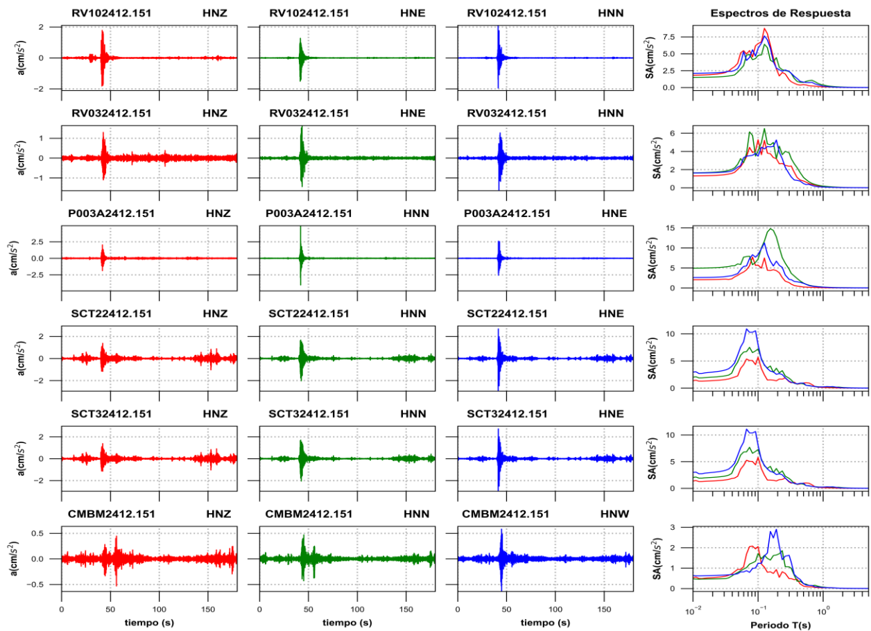
Figura 3a. Acelerogramas registrados y espectros de respuesta estimados para los registros obtenidos durante el sismo del 15 de diciembre de 2024 (M2.2)
