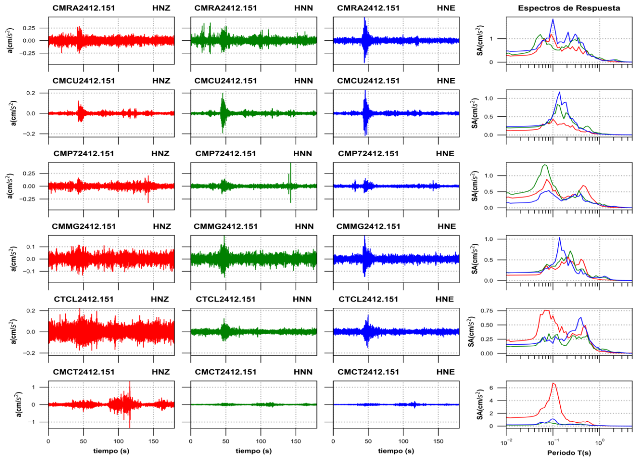
Figura 3c. Acelerogramas registrados y espectros de respuesta estimados para los registros obtenidos durante el sismo del 15 de diciembre de 2024 (M2.2)
