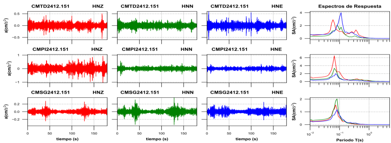
Figura 3f. Acelerogramas registrados y espectros de respuesta estimados para los registros obtenidos durante el sismo del 15 de diciembre de 2024 (M2.2)
