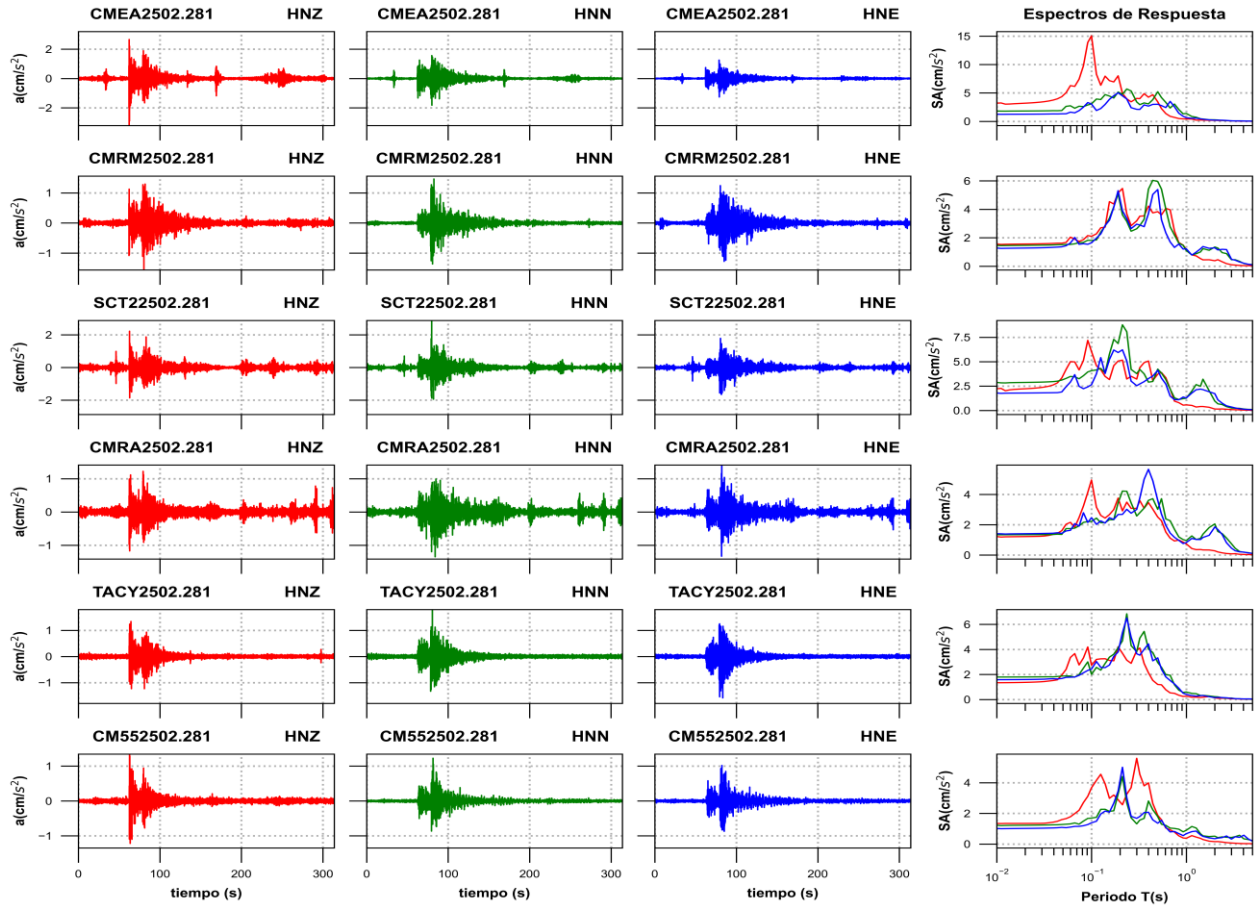
Figura 3c. Acelerogramas registrados y espectros de respuesta estimados para los registros obtenidos durante el sismo del 28 de febrero de 2025 (M5.1)
