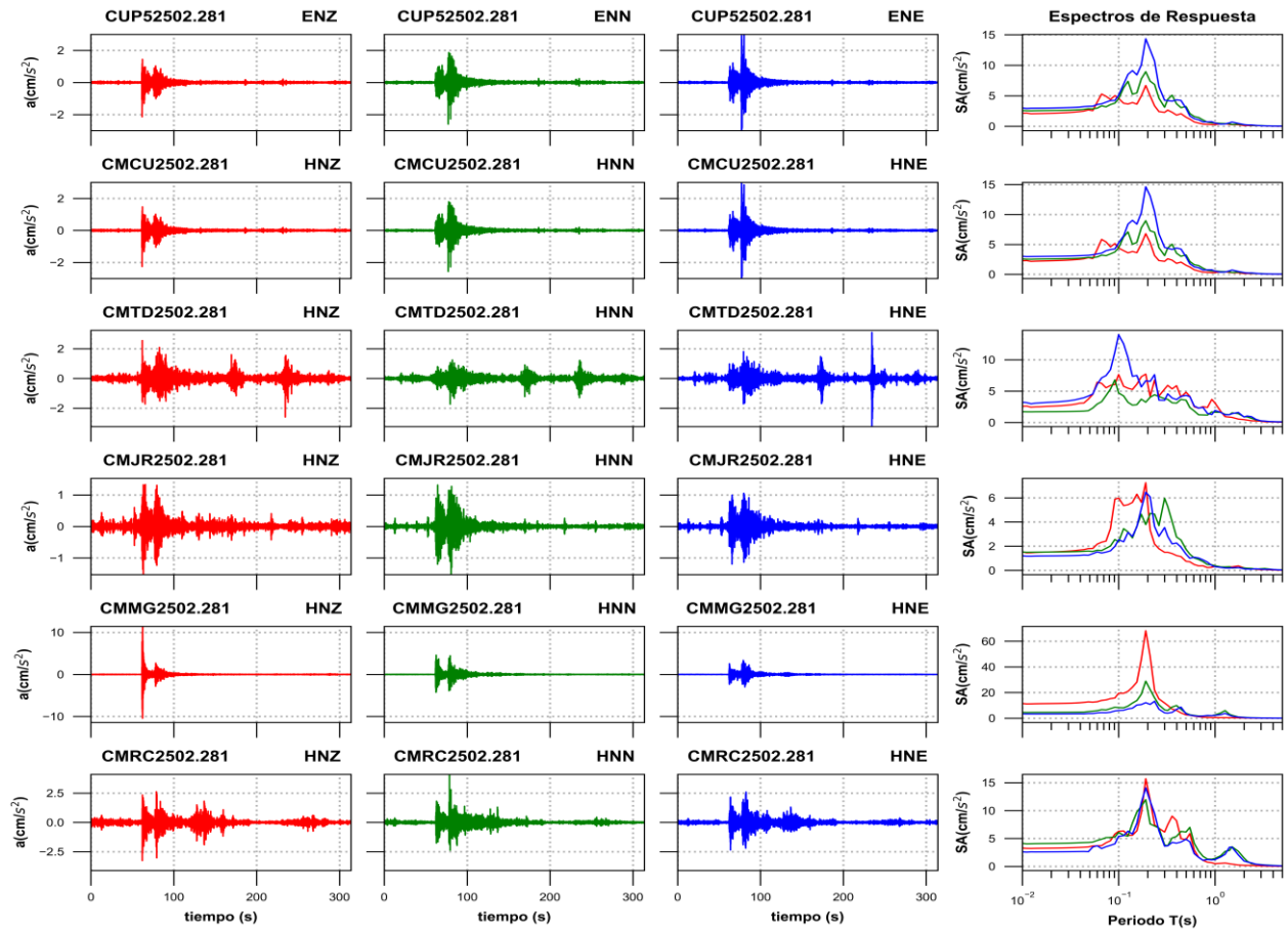
Figura 3b. Acelerogramas registrados y espectros de respuesta estimados para los registros obtenidos durante el sismo del 28 de febrero de 2025 (M5.1)
