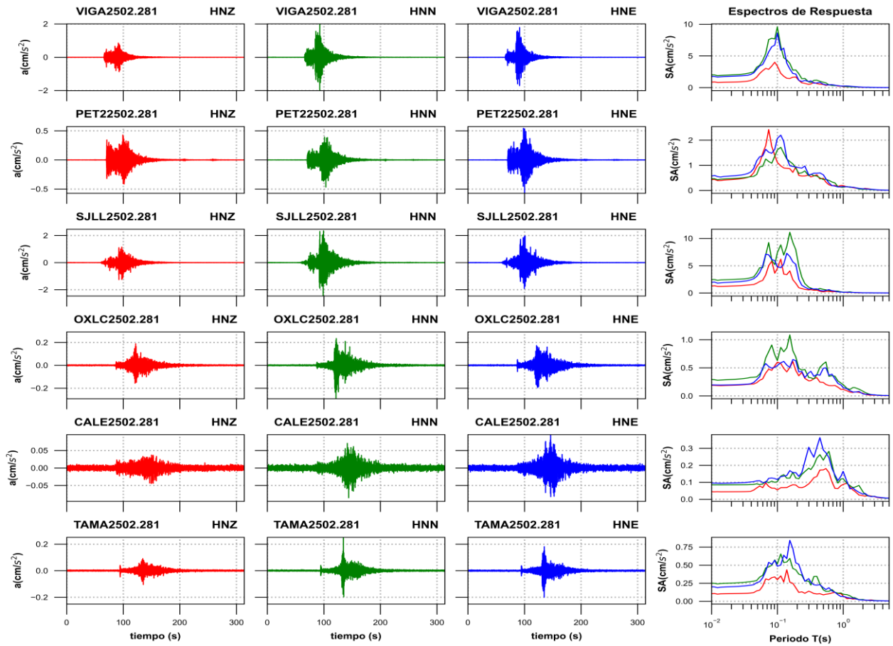
Figura 3f. Acelerogramas registrados y espectros de respuesta estimados para los registros obtenidos durante el sismo del 28 de febrero de 2025 (M5.1)
