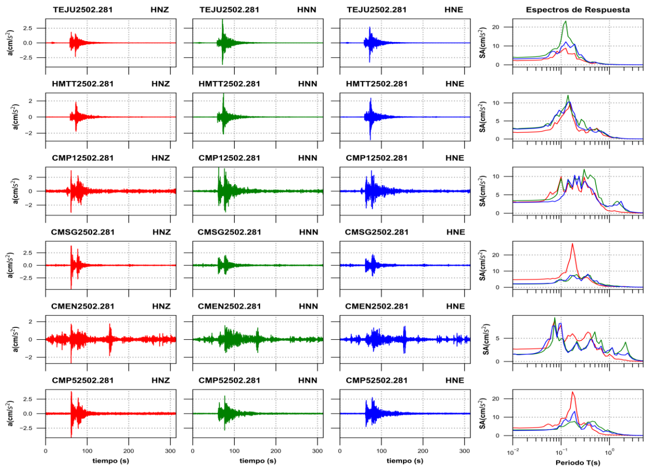
Figura 3a. Acelerogramas registrados y espectros de respuesta estimados para los registros obtenidos durante el sismo del 28 de febrero de 2025 (M5.1)
