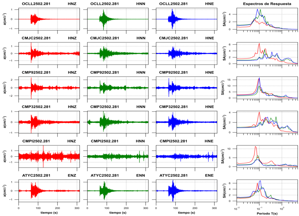
Figura 3e. Acelerogramas registrados y espectros de respuesta estimados para los registros obtenidos durante el sismo del 28 de febrero de 2025 (M5.1)
