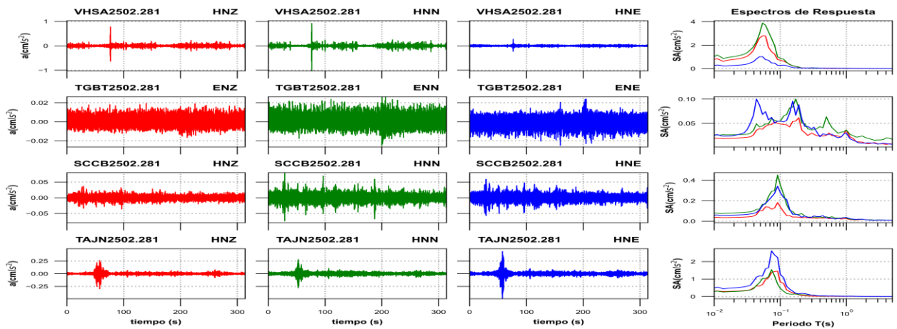
Figura 3h. Acelerogramas registrados y espectros de respuesta estimados para los registros obtenidos durante el sismo del 28 de febrero de 2025 (M5.1)
