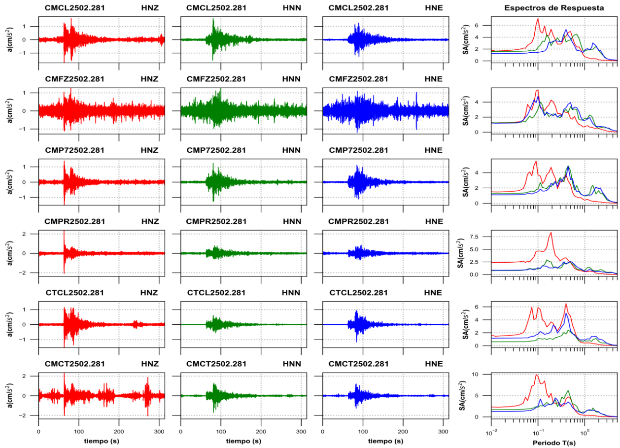
Figura 3d. Acelerogramas registrados y espectros de respuesta estimados para los registros obtenidos durante el sismo del 28 de febrero de 2025 (M5.1)
