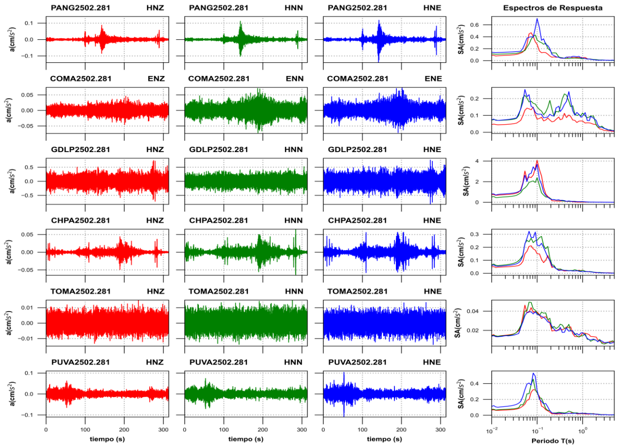
Figura 3g. Acelerogramas registrados y espectros de respuesta estimados para los registros obtenidos durante el sismo del 28 de febrero de 2025 (M5.1)
