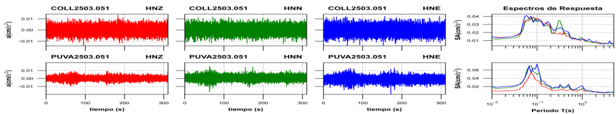
Figura 3h. Acelerogramas registrados y espectros de respuesta estimados para los registros obtenidos durante el sismo del 05 de marzo de 2025 (M5.4)
