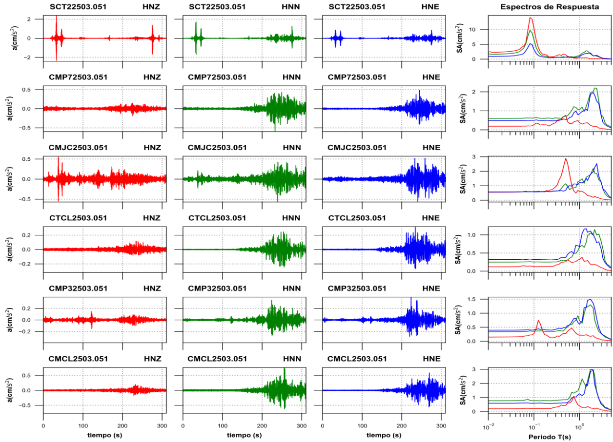
Figura 3f. Acelerogramas registrados y espectros de respuesta estimados para los registros obtenidos durante el sismo del 05 de marzo de 2025 (M5.4)
