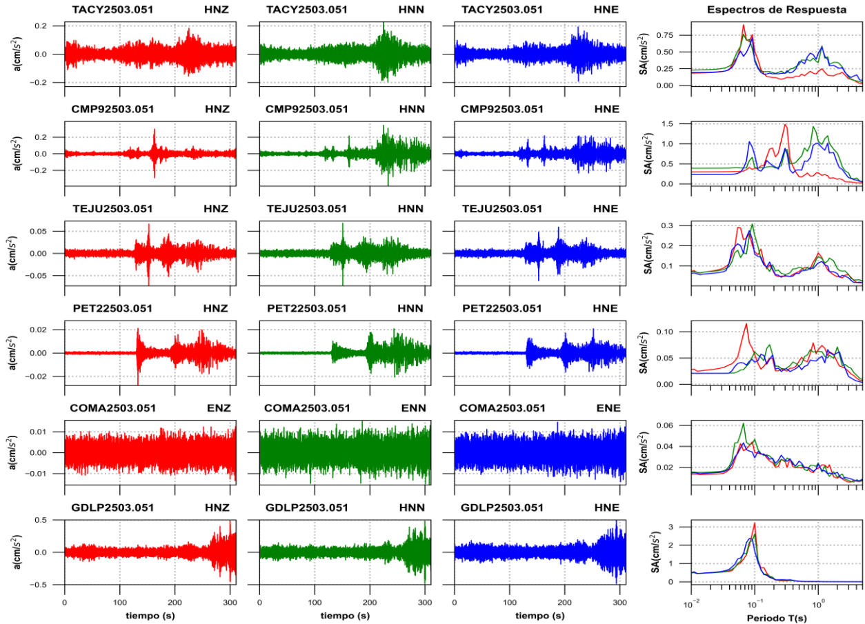
Figura 3g. Acelerogramas registrados y espectros de respuesta estimados para los registros obtenidos durante el sismo del 05 de marzo de 2025 (M5.4)
