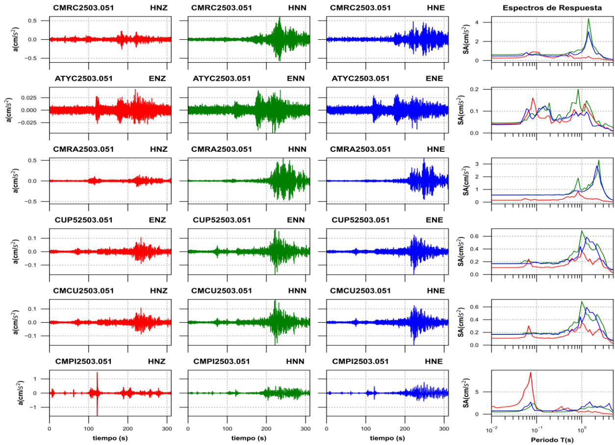
Figura 3e. Acelerogramas registrados y espectros de respuesta estimados para los registros obtenidos durante el sismo del 05 de marzo de 2025 (M5.4)
