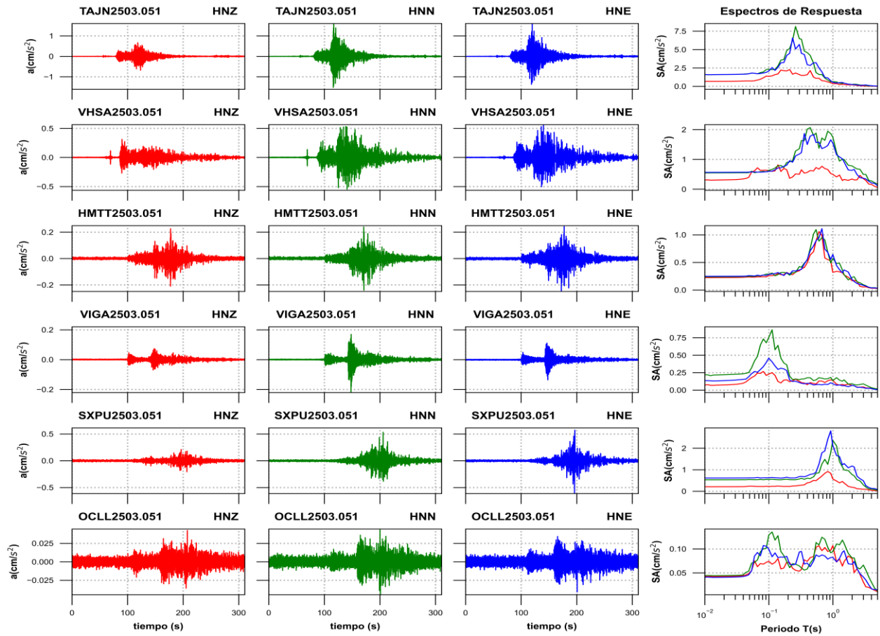
Figura 3b. Acelerogramas registrados y espectros de respuesta estimados para los registros obtenidos durante el sismo del 05 de marzo de 2025 (M5.4)
