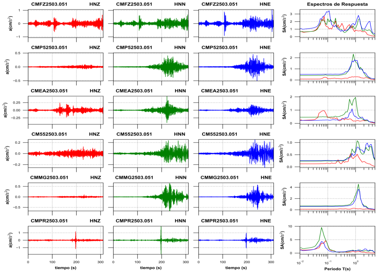
Figura 3d. Acelerogramas registrados y espectros de respuesta estimados para los registros obtenidos durante el sismo del 05 de marzo de 2025 (M5.4)
