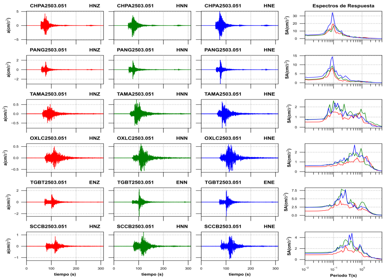
Figura 3a. Acelerogramas registrados y espectros de respuesta estimados para los registros obtenidos durante el sismo del 05 de marzo de 2025 (M5.4)
