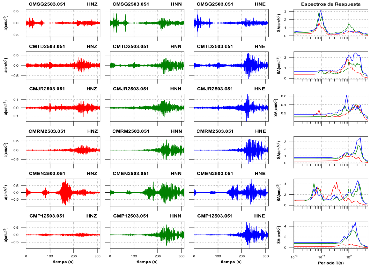
Figura 3c. Acelerogramas registrados y espectros de respuesta estimados para los registros obtenidos durante el sismo del 05 de marzo de 2025 (M5.4)
